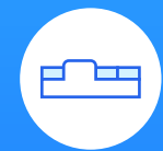
리본(Ribbon) UI
